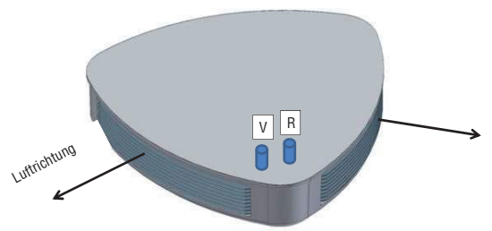
Darstellung PWW Anschlüsse Luftrichtung von unten, seitlich ausblasend
