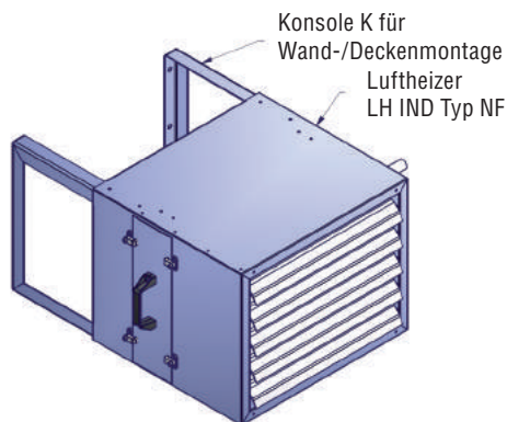
Wandmontage LH IND Typ NF
