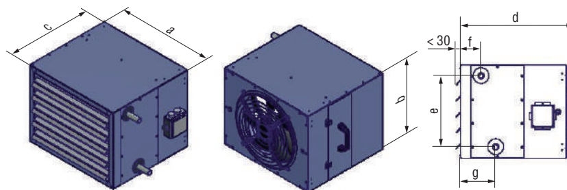
Abb.: Geräteserie Typ LH...-HF
