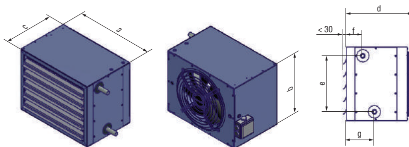
Abb.: Geräteserie Typ LH...-H
