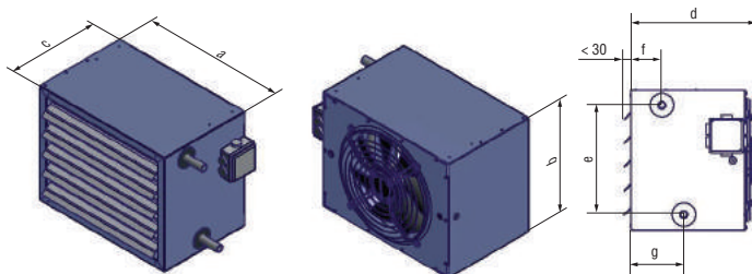
Abb.: Geräteserie Typ LH...-N
