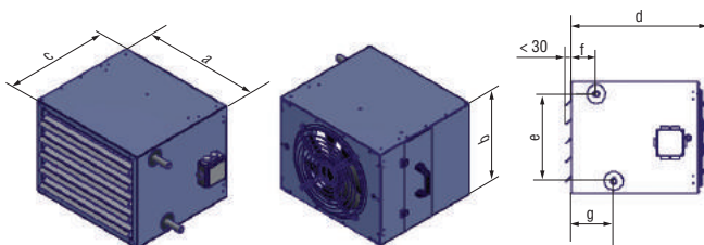
Abb.: Geräteserie Typ LH...-NF
