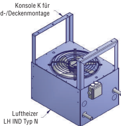
Deckenmontage LH IND Typ N
